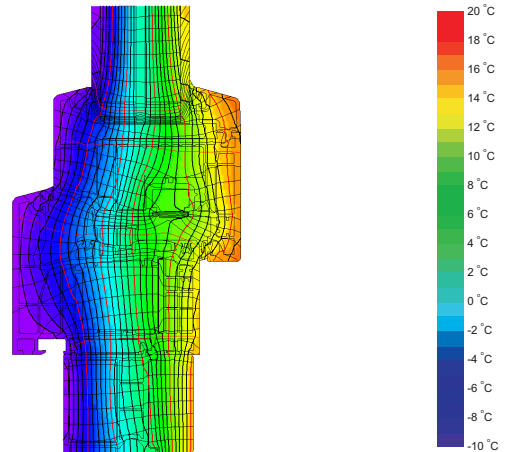
Isothermengrafik
