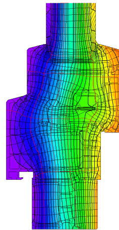
Isothermengrafik
