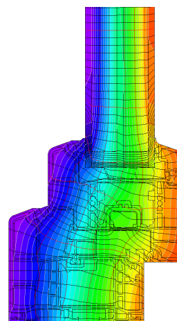
Isothermengrafik
