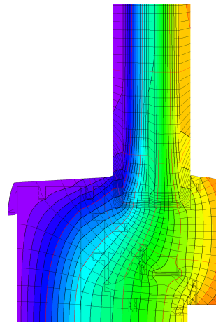
Isothermengrafik
