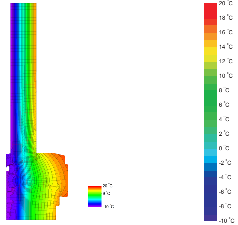
Isothermengrafik
