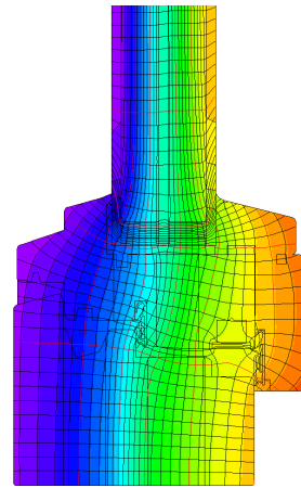
Isothermengrafik
