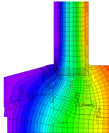
Isothermengrafik
