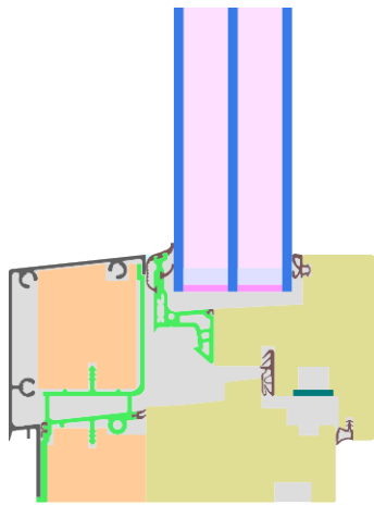
Berechnungsmodell
