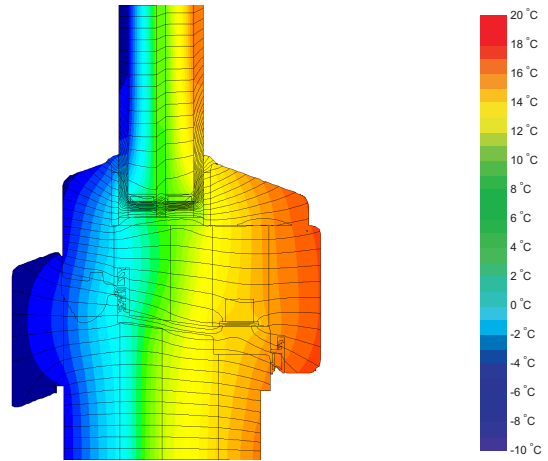
Isothermengrafik
