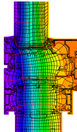
Isothermengrafik
