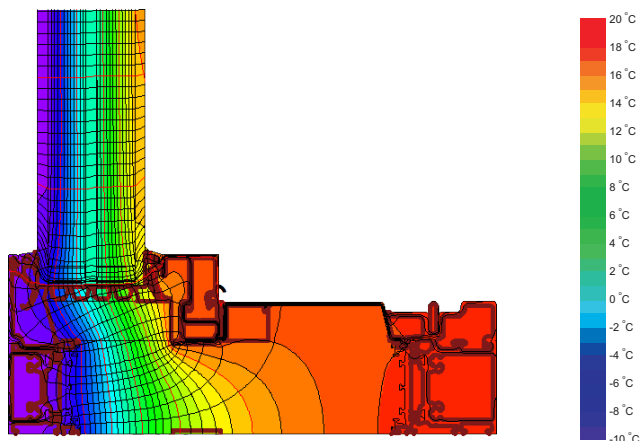
Isothermengrafik
