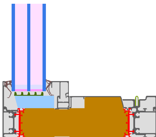
Berechnungsmodell
