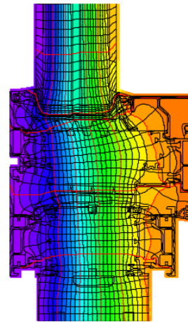
Isothermengrafik
