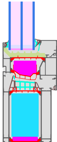
Berechnungsmodell
