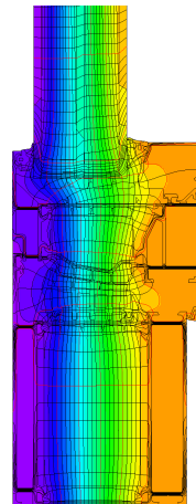
Isothermengrafik
