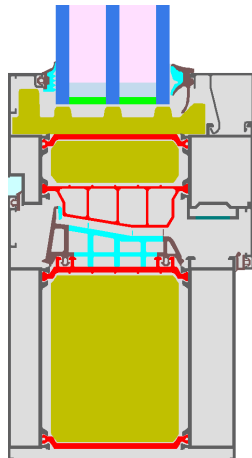
Berechnungsmodell
