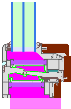
Berechnungsmodell
