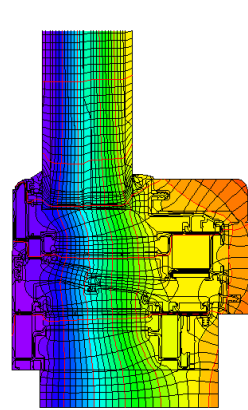
Isothermengrafik
