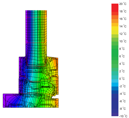
Isothermengrafik
