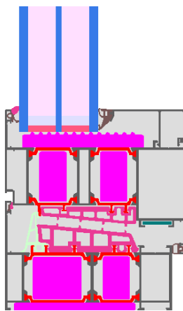
Berechnungsmodell
