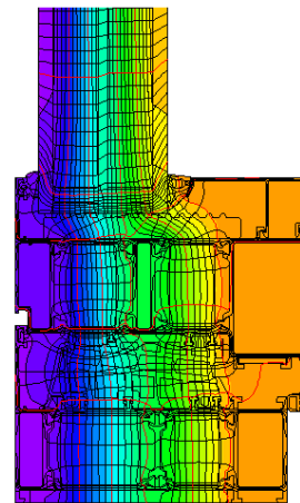
Isothermengrafik
