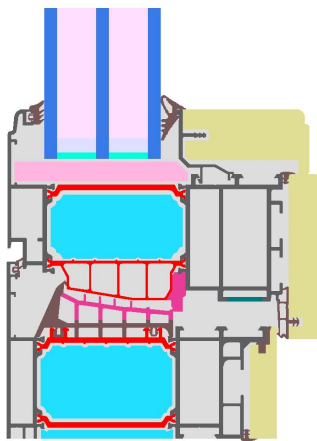
Berechnungsmodell
