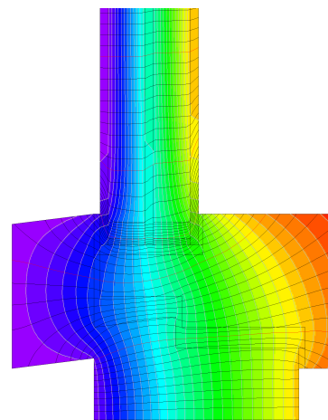
Isothermengrafik
