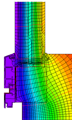
Isothermengrafik
