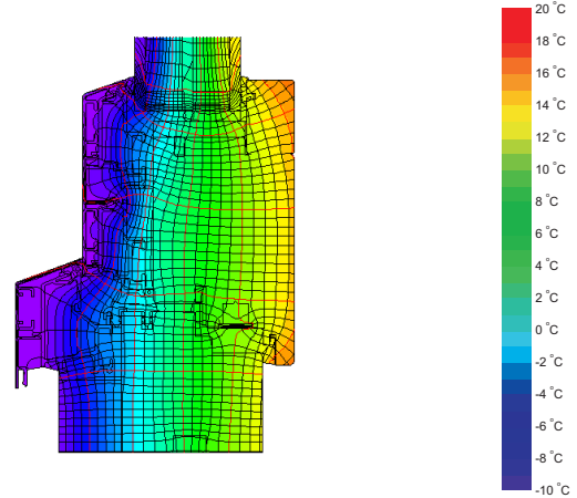
Isothermengrafik
