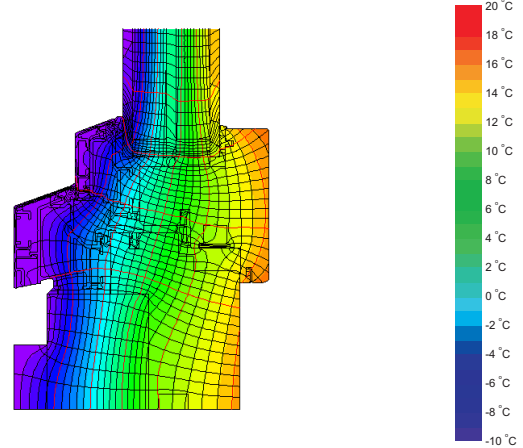
Isothermengrafik
