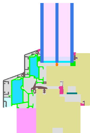
Berechnungsmodell
