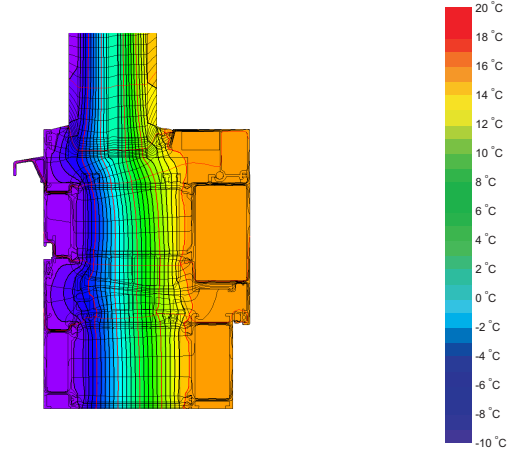
Isothermengrafik
