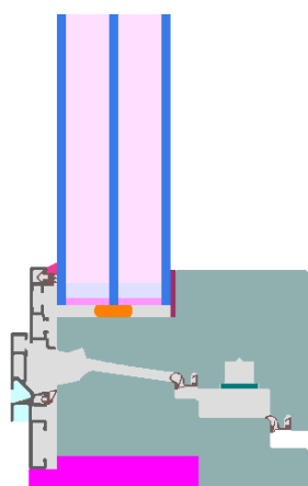
Berechnungsmodell
