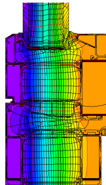
Isothermengrafik
