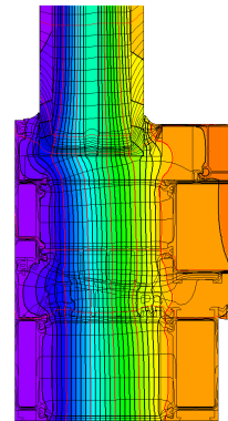
Isothermengrafik
