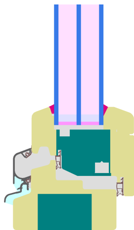
Berechnungsmodell
