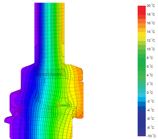
Isothermengrafik
