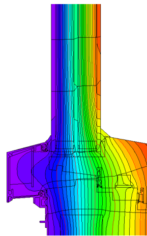
Isothermengrafik
