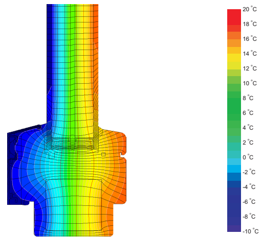
Isothermengrafik
