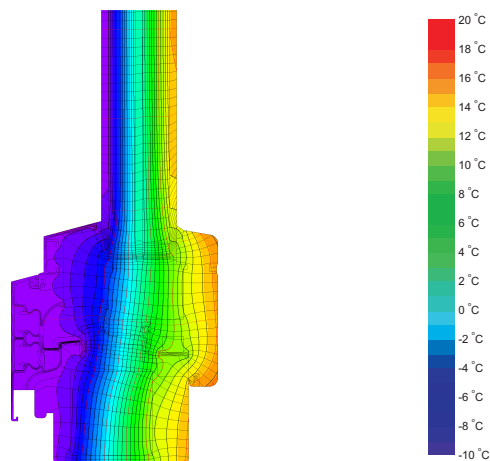
Isothermengrafik
