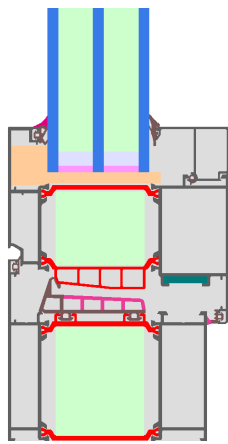
Berechnungsmodell
