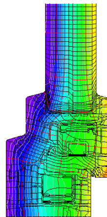
Isothermengrafik
