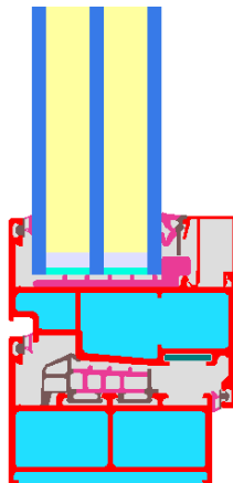
Berechnungsmodell
