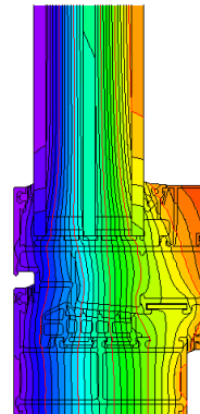
Isothermengrafik
