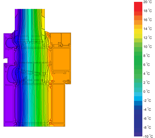
Isothermengrafik
