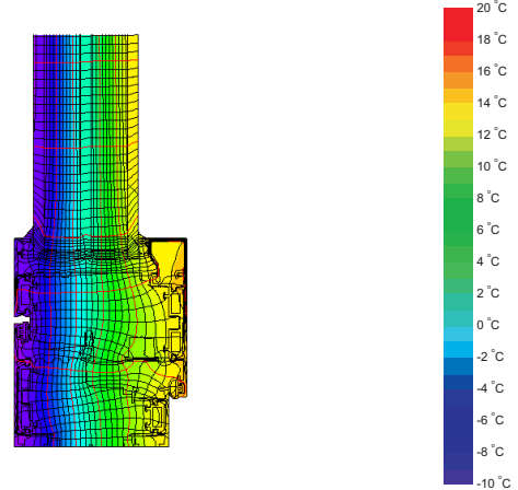
Isothermengrafik
