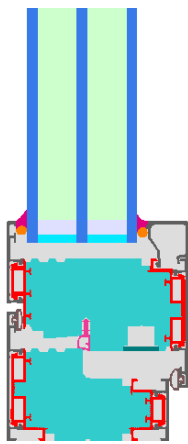
Berechnungsmodell
