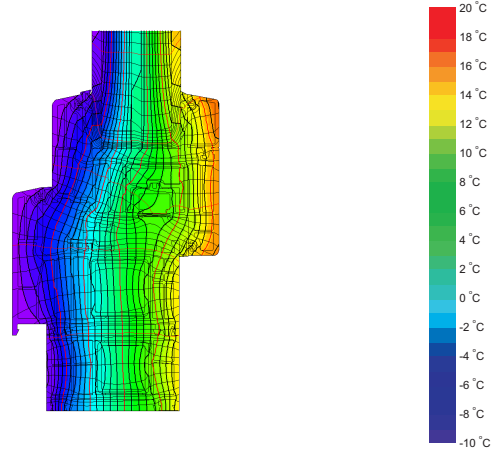
Isothermengrafik
