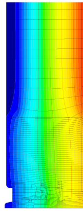
Isothermengrafik
