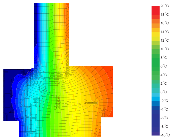
Isothermengrafik
