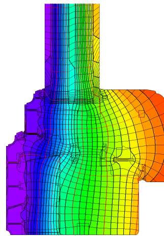
Isothermengrafik
