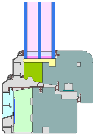
Berechnungsmodell
