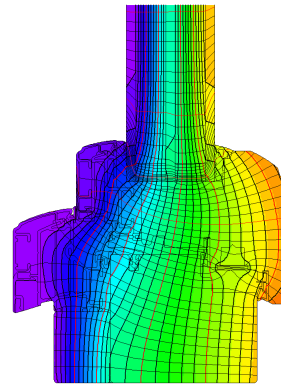
Isothermengrafik
