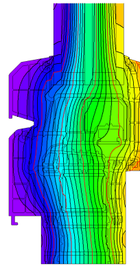
Isothermengrafik
