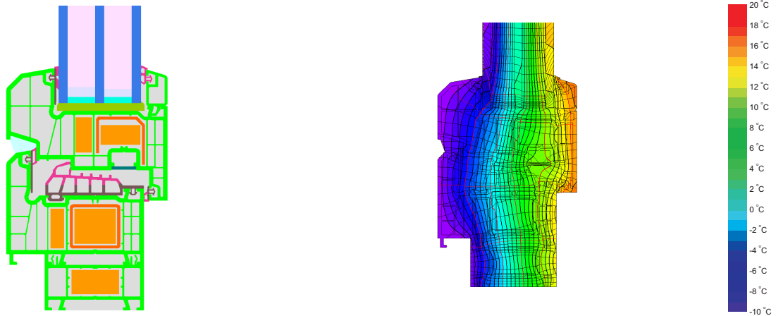
Berechnungsmodell
