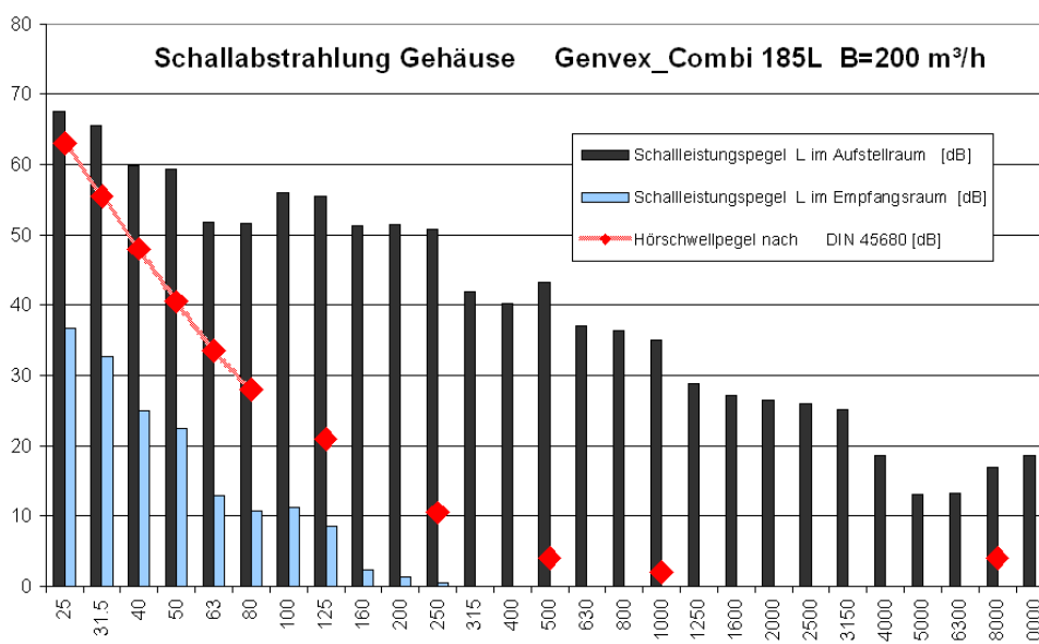
Abbildung 1: Schallabstrahlung des Gehäuses bei Volumenstrom 200 m 3 /h
