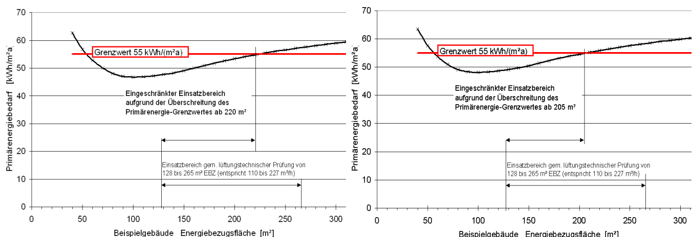
Abbildung 2: Einsatzbereich des Gerätes Genvex 185L, bei Nennvolumenstrom 150 m³/h bzw. 200 m³/h
