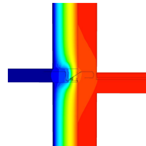
Isothermenbild des XT Typ K-U/K-O-M2V1
