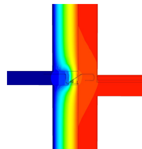
Isothermal map of XT Typ K-U/K-O-M2V1
