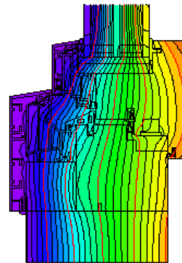
Isothermengrafik
