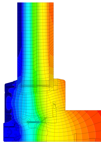
Isothermengrafik
