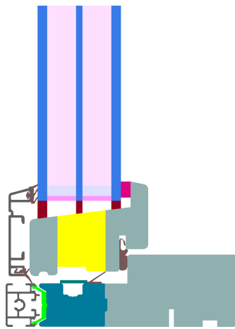
Berechnungsmodell
