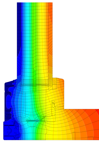
Isothermengrafik
