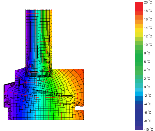
Isothermengrafik
