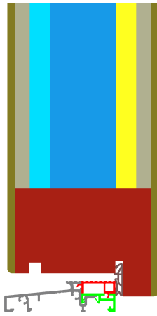
Berechnungsmodell
