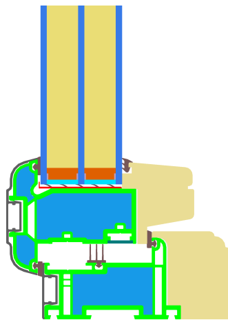
Berechnungsmodell
